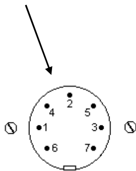
FIGURE 2 Prise DIN femelle J4n (vue de l'arrière du JRC)
