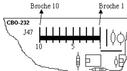
FIGURE 3 Brochage du connecteur J47
