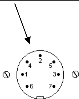
FIGURE 2 Prise DIN femelle J4n (vue de l'arrière du JRC)
